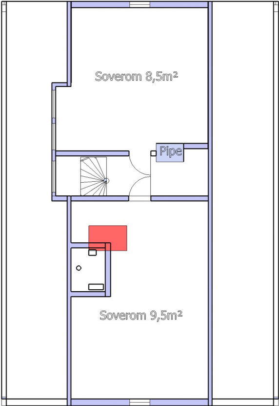
Ny planløsning loft, plassering av nytt takvindu markert i rødt
